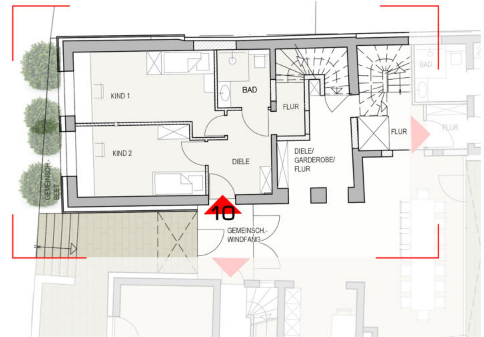
Erdgeschoss
