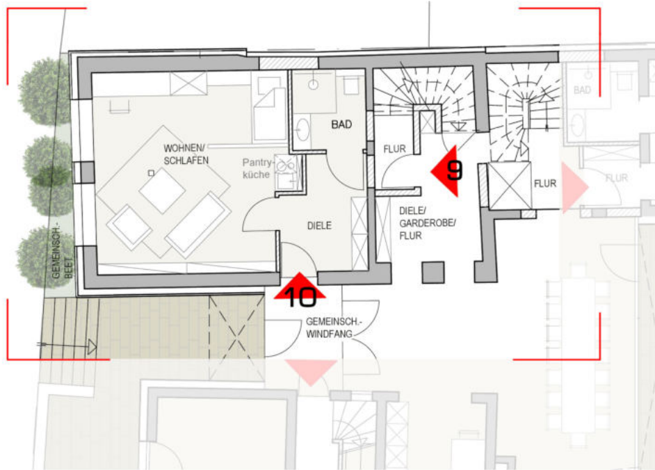
Erdgeschoss
